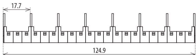
Listwa łącząca CB-17-8
