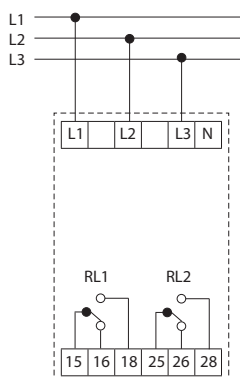
podłączenie 3-przewodowe
