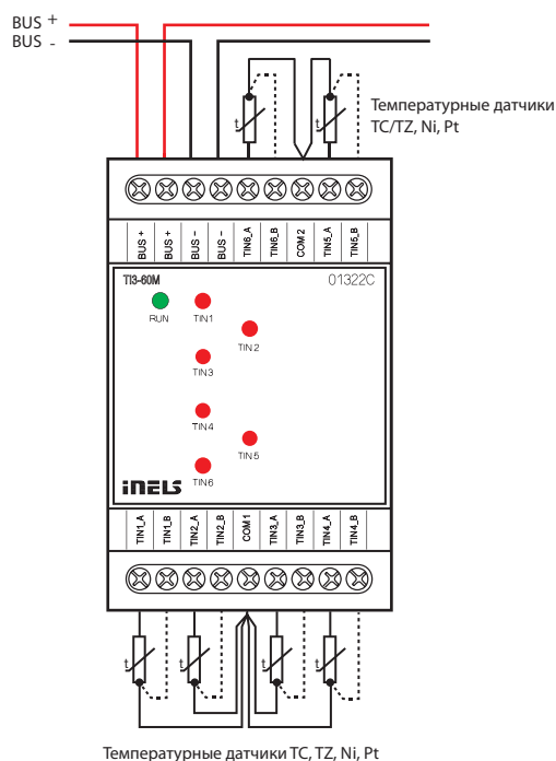
Температурные датчики TC, TZ, Ni, Pt
